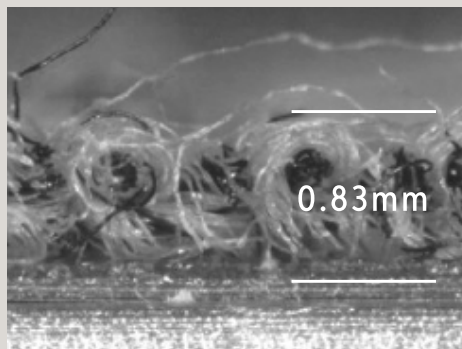
マーフィル®CO 28G天竺断面
